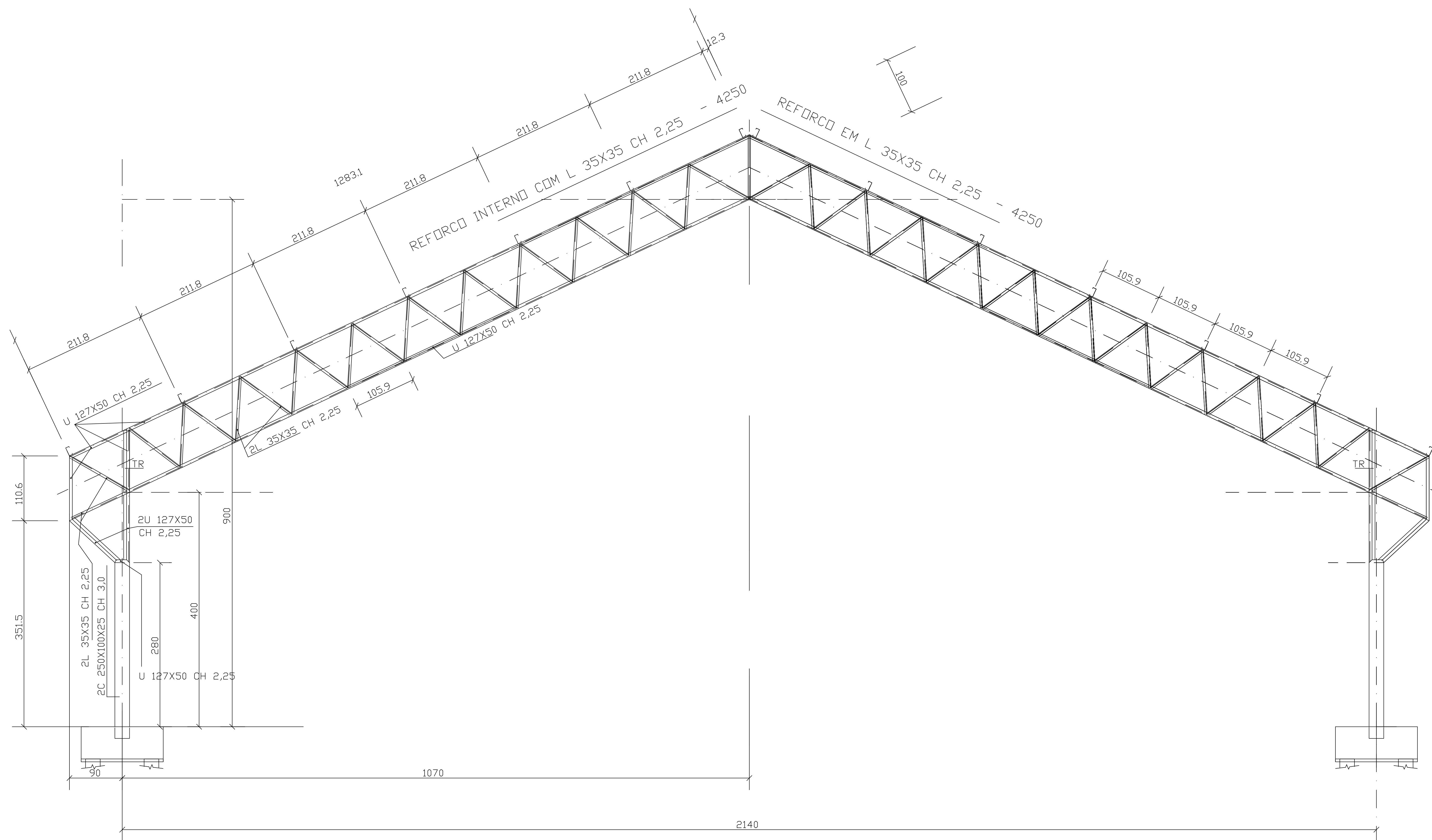
DETALHE PORTICO PRINCIPAL ( X7 )
