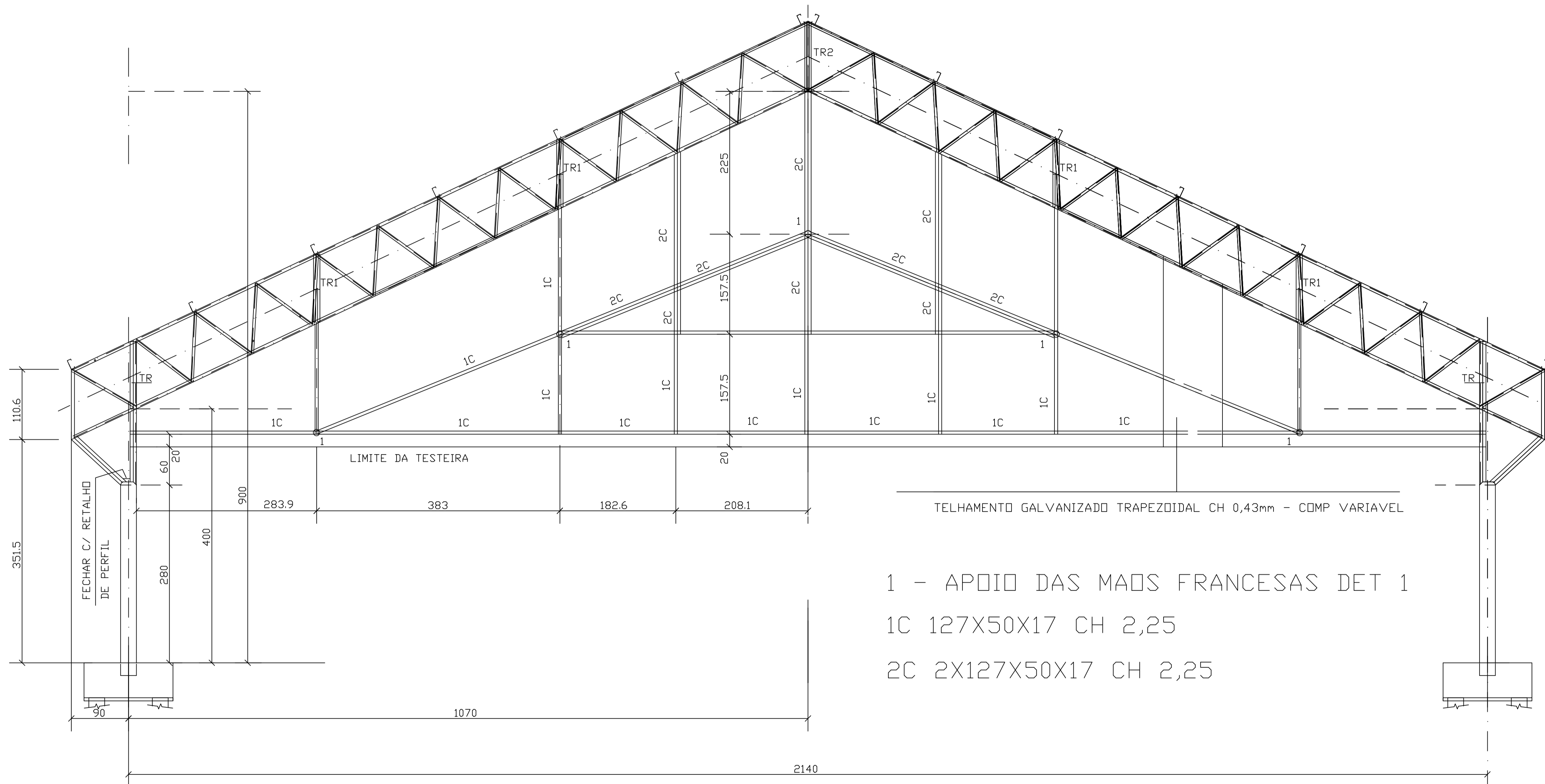
DETALHE DO PÓRTICO EXTREMO ( X2 )
